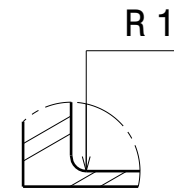
DETALLE C ESCALA: 2:1
