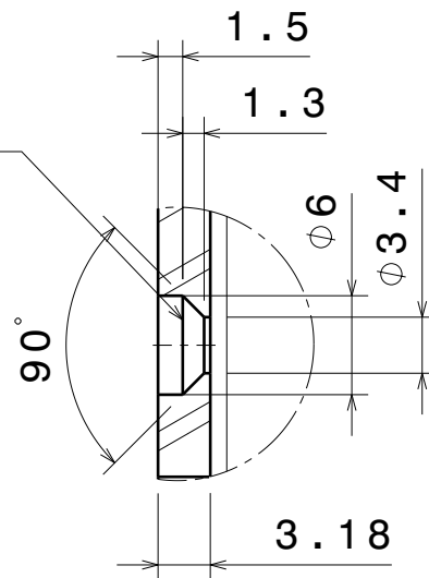
DETALLE B ESCALA: 2:1
